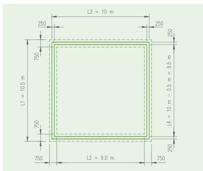
FIGURE 1 Dimension du mur (vue en plan)
