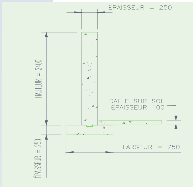
FIGURE 2 Dimension de la semelle et du mur (vue en coupe)
