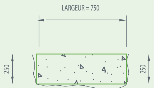
FIGURE 3 Irrégularités de la semelle
